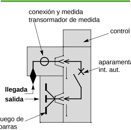
Fig. 17: Los distintos compartimentos de una celda de MT, bajo envolvente metálica, y sus principales elementos.
