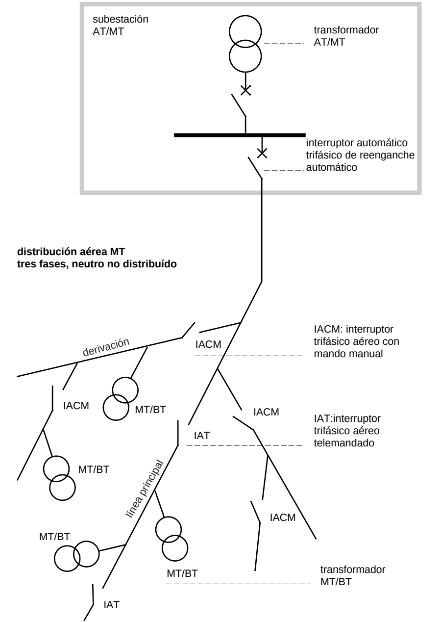
Fig. 20: Esquema de distribución aérea de MT. (EDF - Francia).
