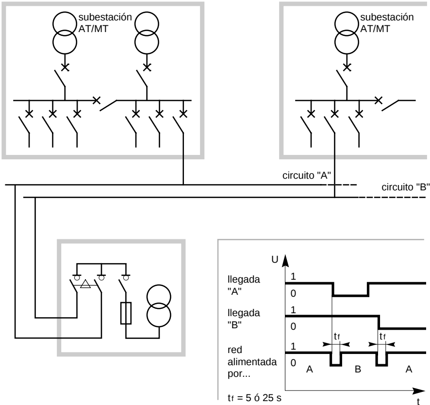
Fig. 11: Esquema de distribución en doble derivación, utilizado por EDF-Francia. En el recuadro, secuencia del automatismo de un permutador Merlin Gerin, conforme con las especificaciones EDF-Francia.
