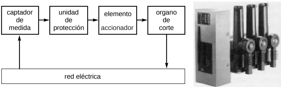
Fig. 14: Cadena de protección de MT, y fotografía de un SF Set (Merlin Gerin), un ejemplo de integración completa.
